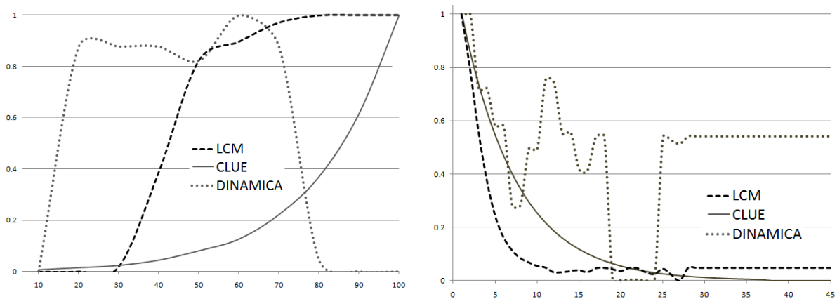
Figura 3. Probabilidad de cambio en función de la elevación (izquierda) y la distancia a la carretera (derecha).
